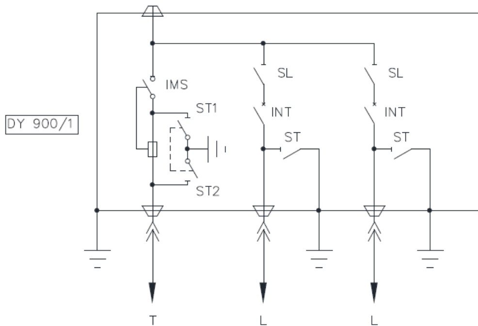
Figura G-12 Schema di principio nella configurazione 2LEi+1T (DY900/1) – lato MEGARETI.
