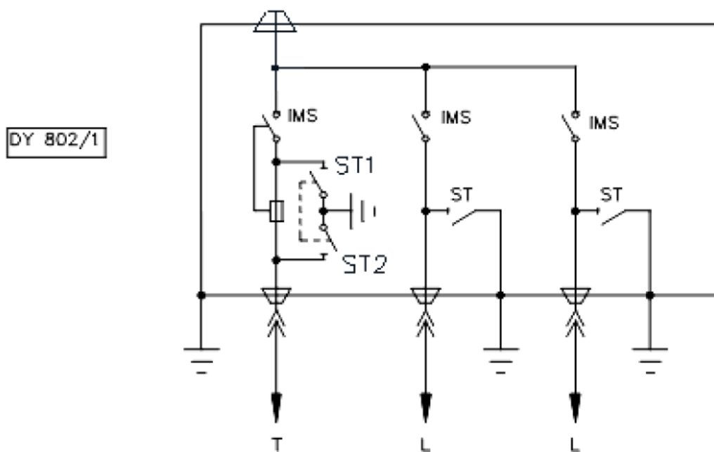
Figura G-13 Schema di principio nella configurazione 2LE+1T (DY802/1) – lato MEGARETI.
