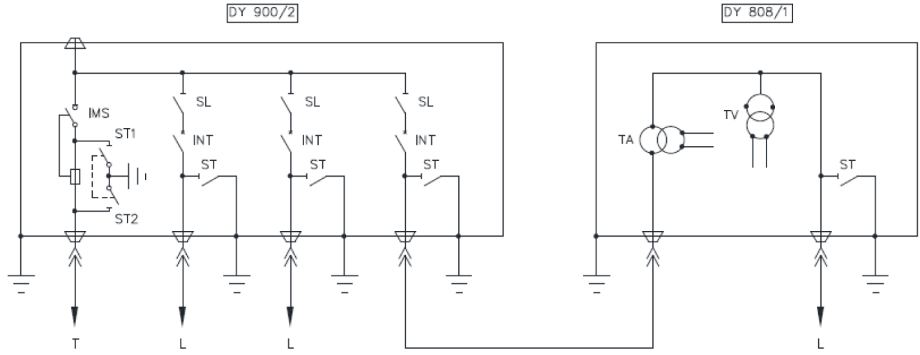
Figura G-15 Esempio schema sinottico lato MEGARETI + lato Cliente.
