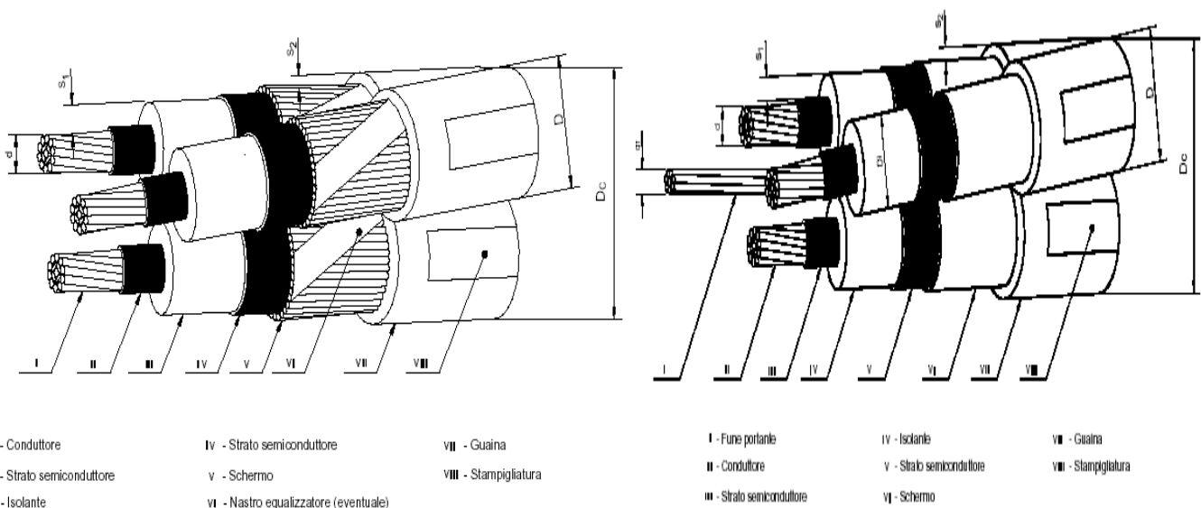
Figura G-7 Composizione dei cavi unificati MEGARETI di impiego prevalente Le sezioni normalizzate sono riportate nella Tabella G-3 e nella Tabella G-4.
