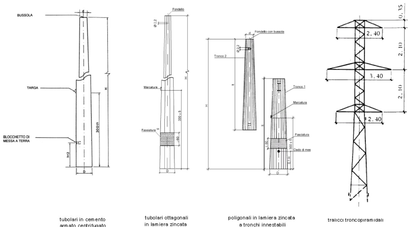
Figura G-8 Caratteristiche dei sostegni unificati MEGARETI di uso prevalente
